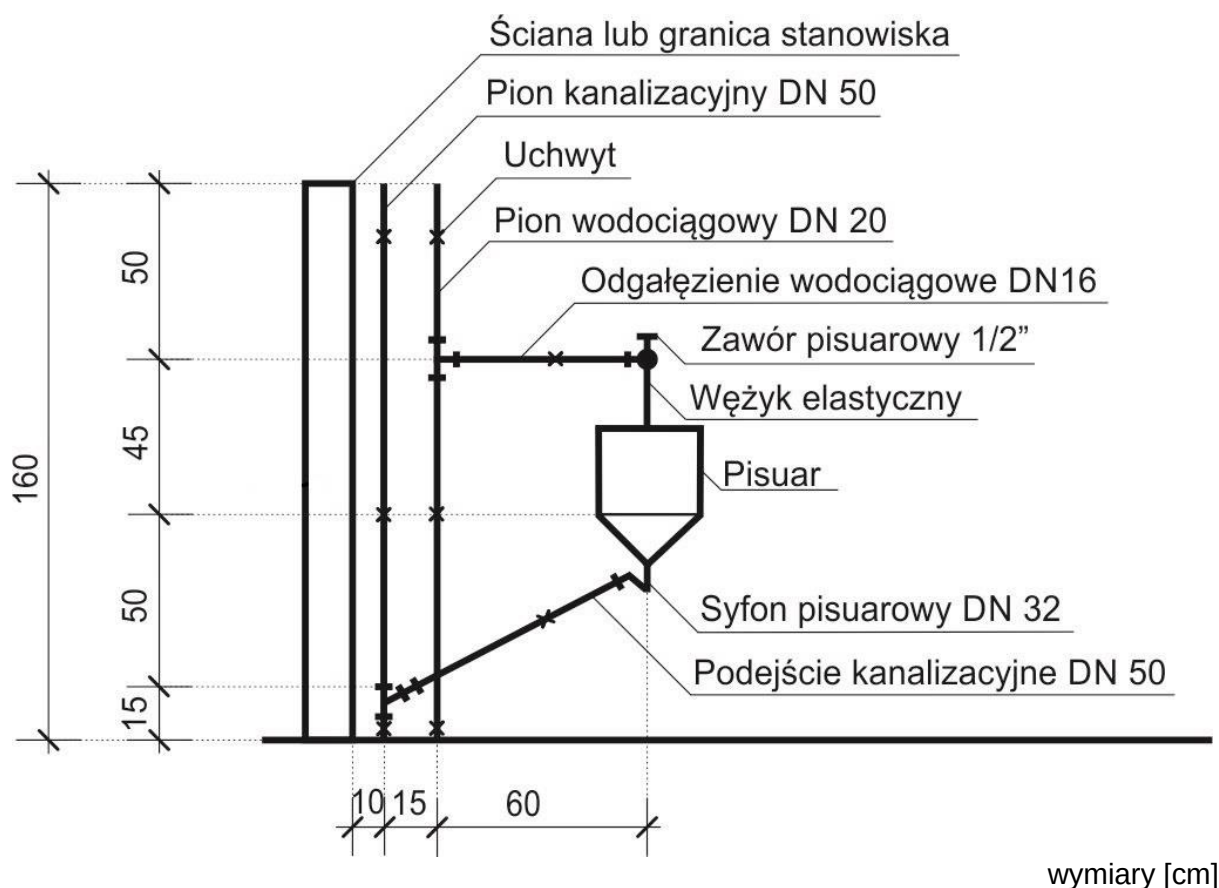
Rysunek 1. Widok pisuaru oraz instalacji wodociągowej i kanalizacyjnej
