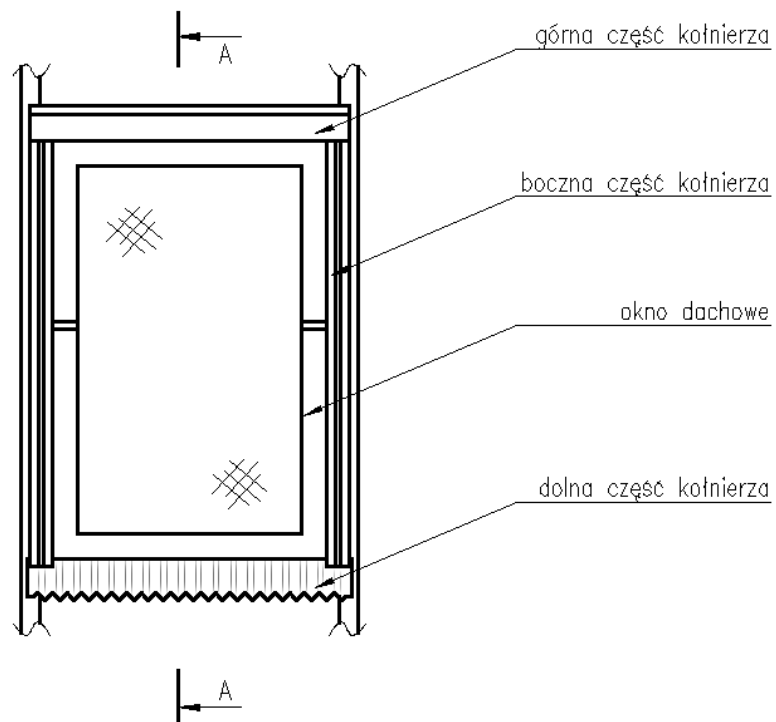
Rysunek 2. Zamontowane okno dachowe z kołnierzem uszczelniającym
