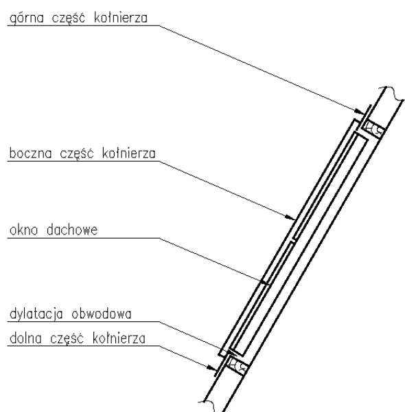
Rysunek 3. Przekrój A-A zamontowanego okna dachowego z kołnierzem uszczelniającym
