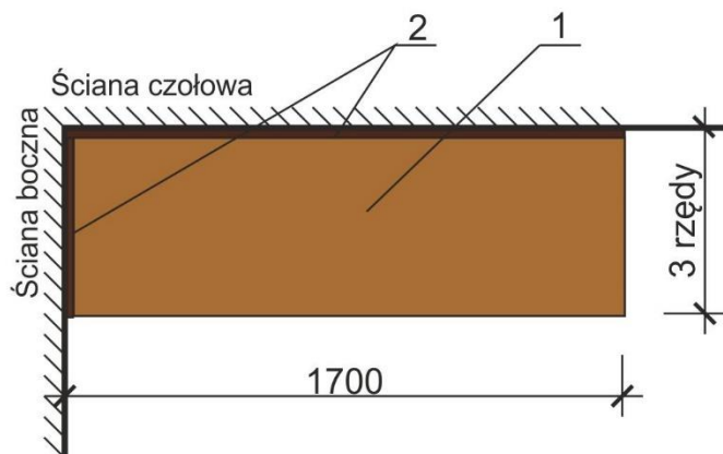
Rzut podłogi
