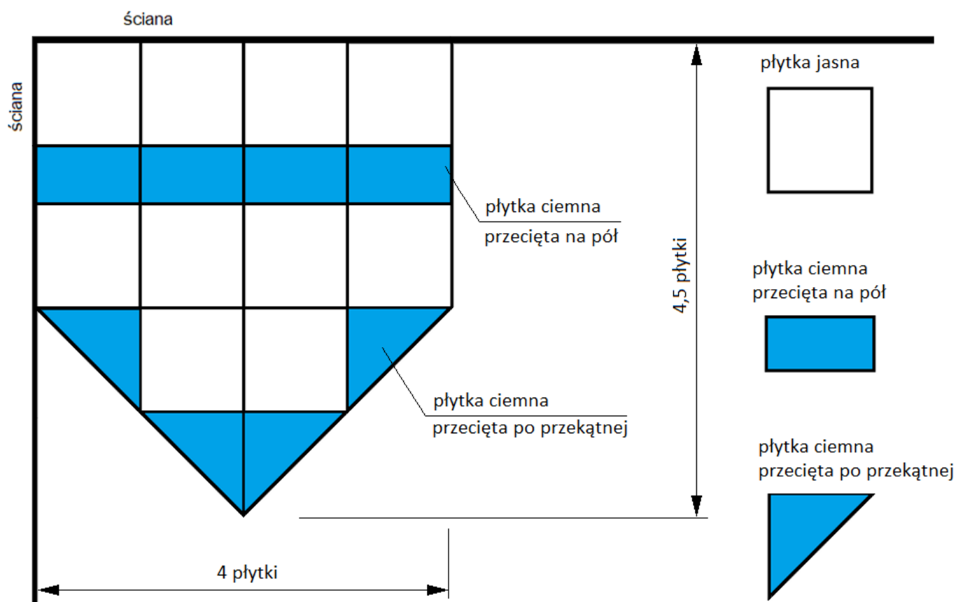
Usytuowanie posadzki na podłożu
