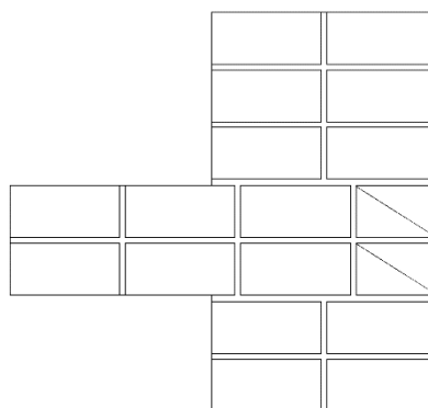
Rysunek 2. Układ cegieł w warstwach przenikających się murów (rzuty)
