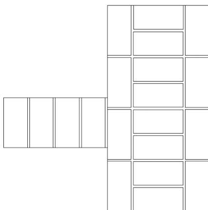
Rysunek 2. Układ cegieł w warstwach przenikających się murów (rzuty)
