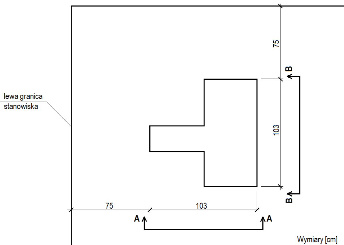
Rysunek 1. Usytuowanie przenikających się murów na stanowisku egzaminacyjnym (rzut)
