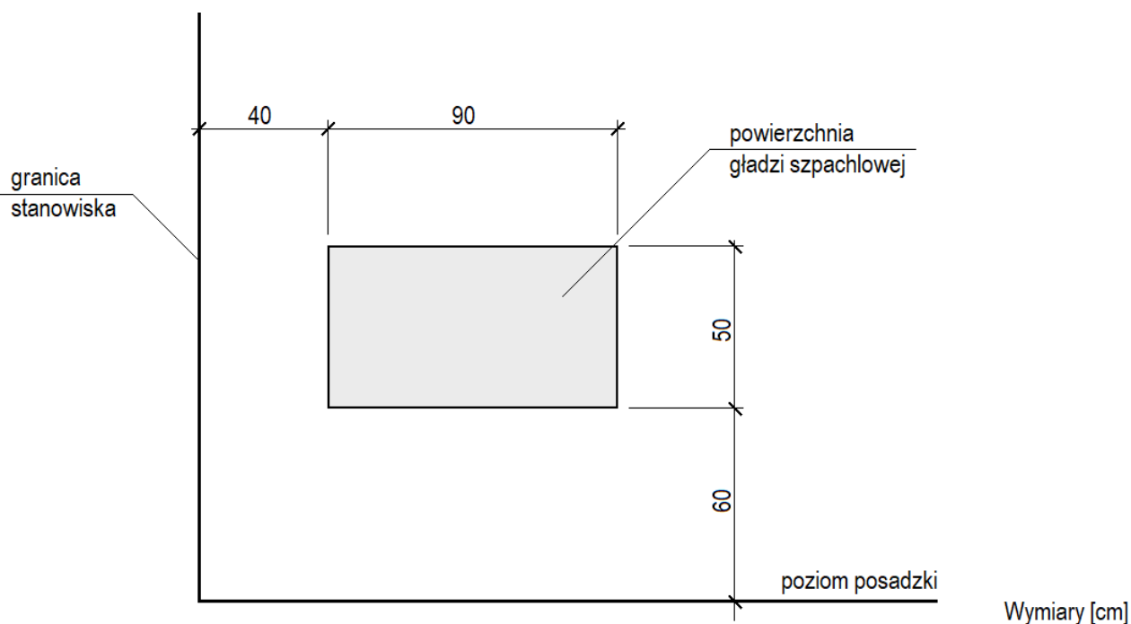
Rysunek 4. Usytuowanie powierzchni gładzi na ścianie stanowiska egzaminacyjnego (widok)
