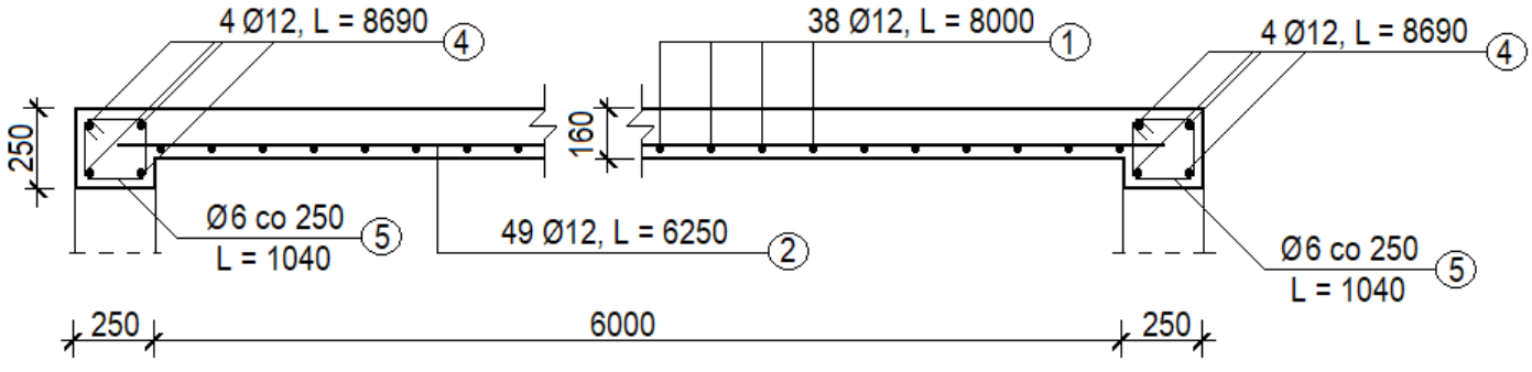
Rysunek konstrukcyjny żelbetowego stropu płytowego i wieńców stropowych – rzut i przekroje
