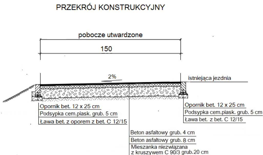
Rysunek 1. Przekrój konstrukcyjny utwardzonego pobocza z jednej strony drogi o prostym odcinku.
