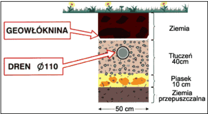
Rysunek 4. Przekrój pionowy przez drenaż rozsączający (warstwy montażowe)
