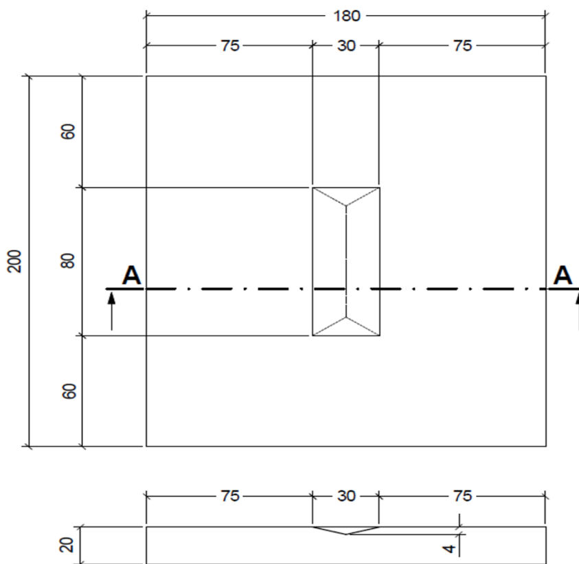
Widok i przekrój A-A płytki z literą I
