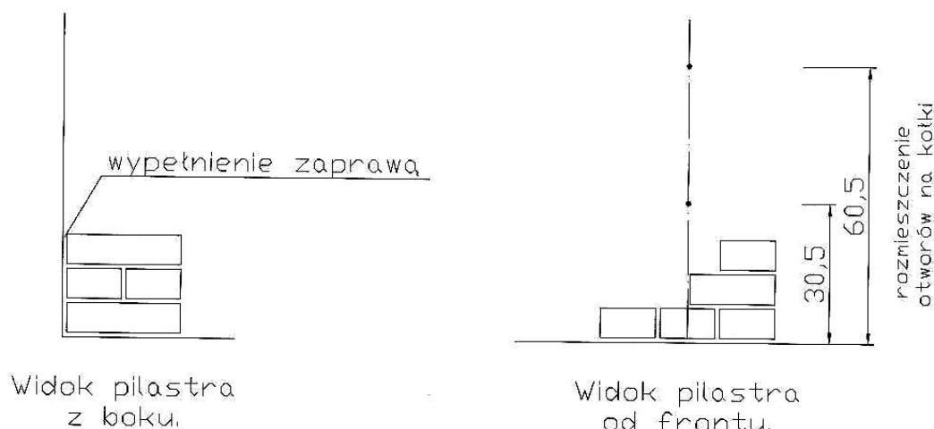
Rysunek 1. Istniejąca baza pilastra
