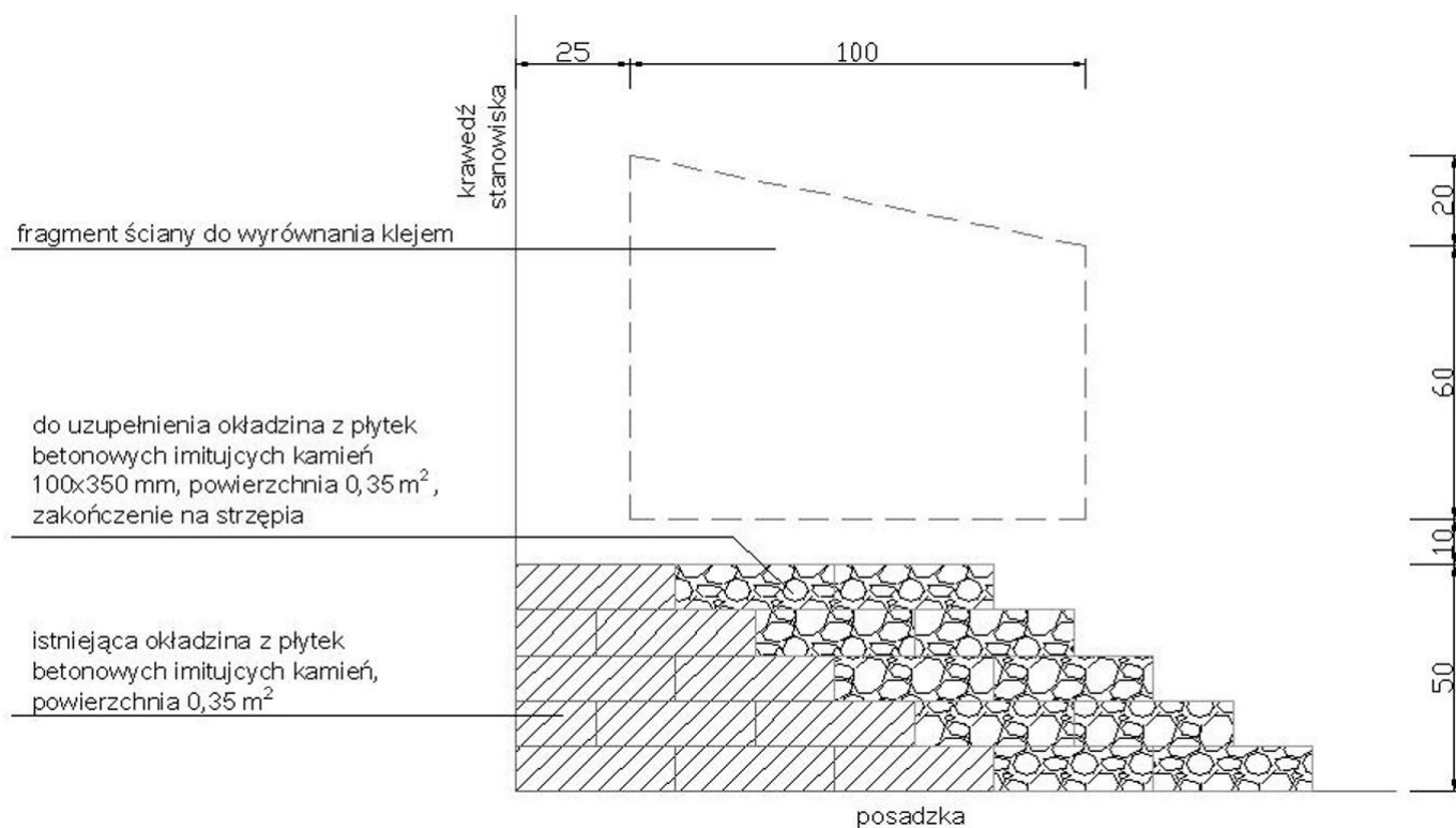
Rysunek. Fragment ściany do wyrównania klejem.
