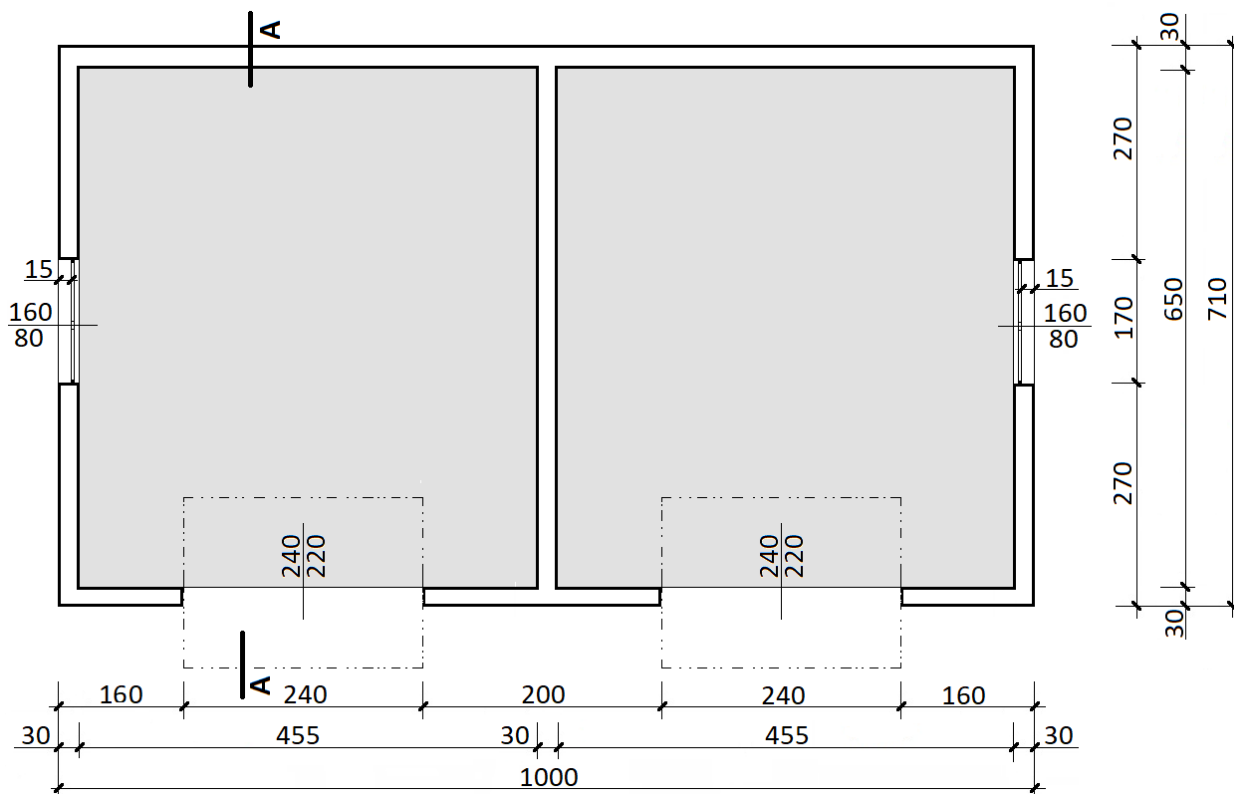
Rysunek 1. Rzut garażu
