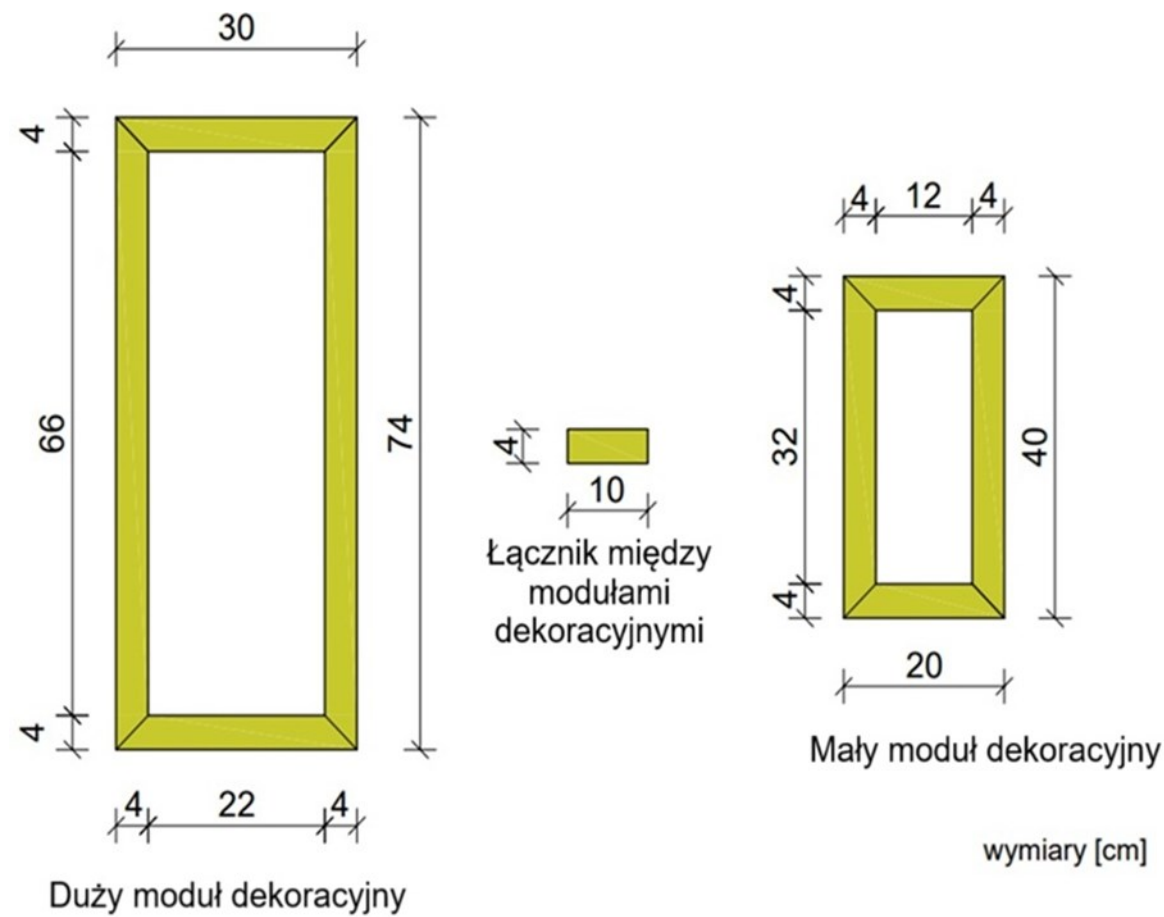
Rysunek 2. Wymiary elementów dekoracji ściennej
