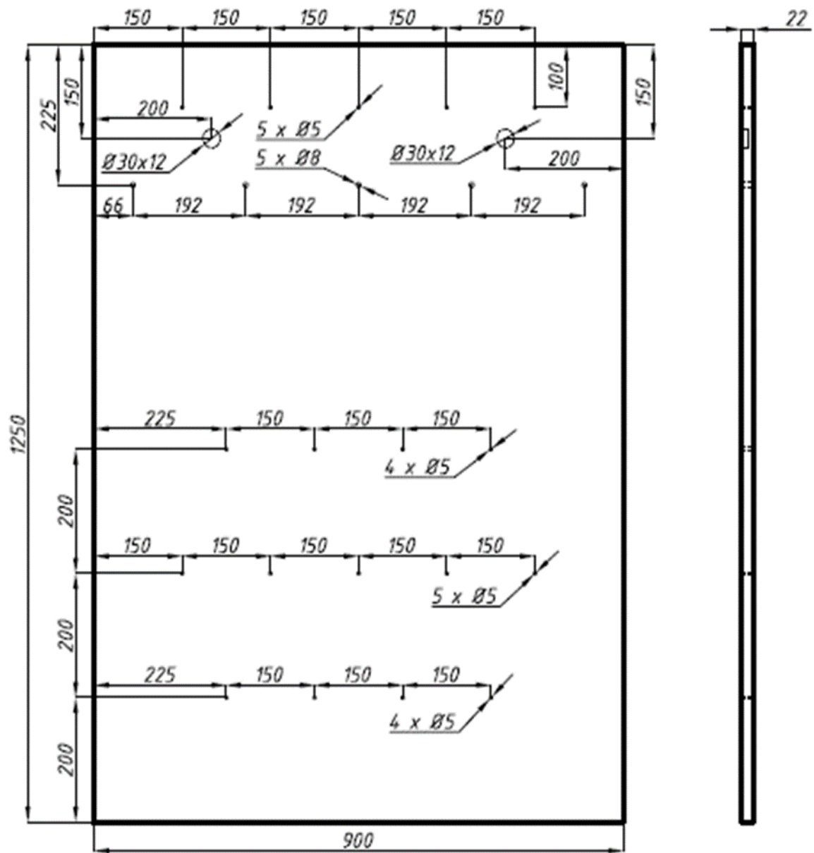
Schemat 1. Płyta panelu ściennego
