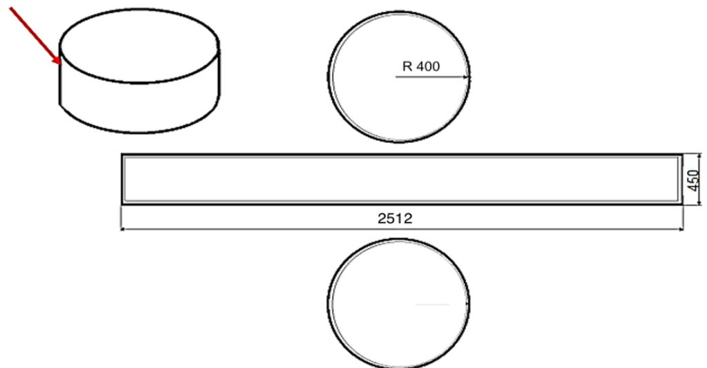
Rysunek 1. Poszewka wewnętrzna pufu kibica
