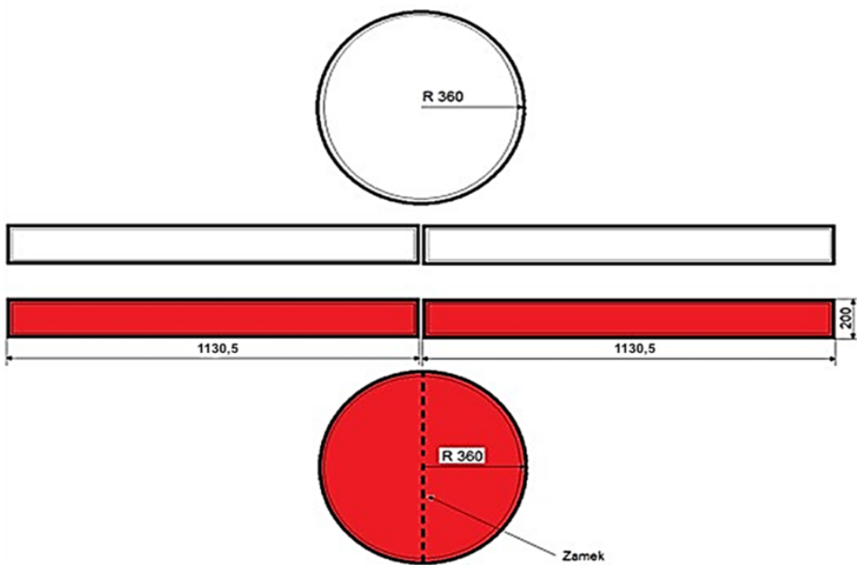
Rysunek 3. Pokrowiec pufu kibica
