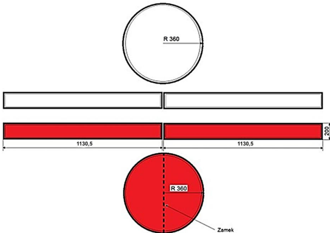
Rysunek 3. Pokrowiec pufu kibica
