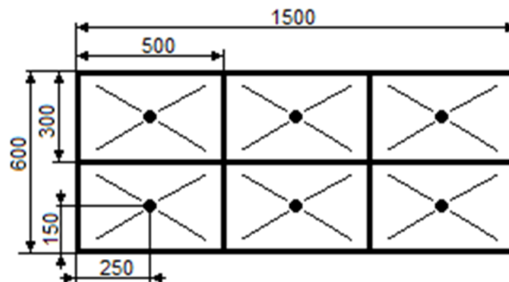
Rysunek 3. Gotowy panel ścienny
