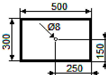
Rysunek 2. Podłoże segmentu panelu
