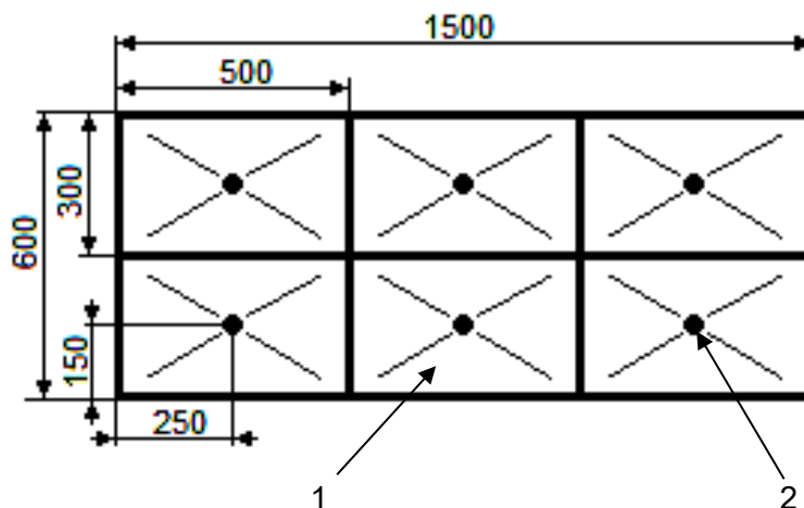
Rysunek 1. Panel ścienny: 1 – segment panelu, 2 – guzik
