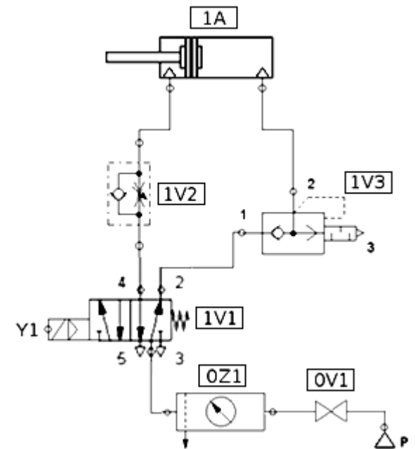
Rys. 2. Schemat połączeń pneumatycznych układu elektropneumatycznego
