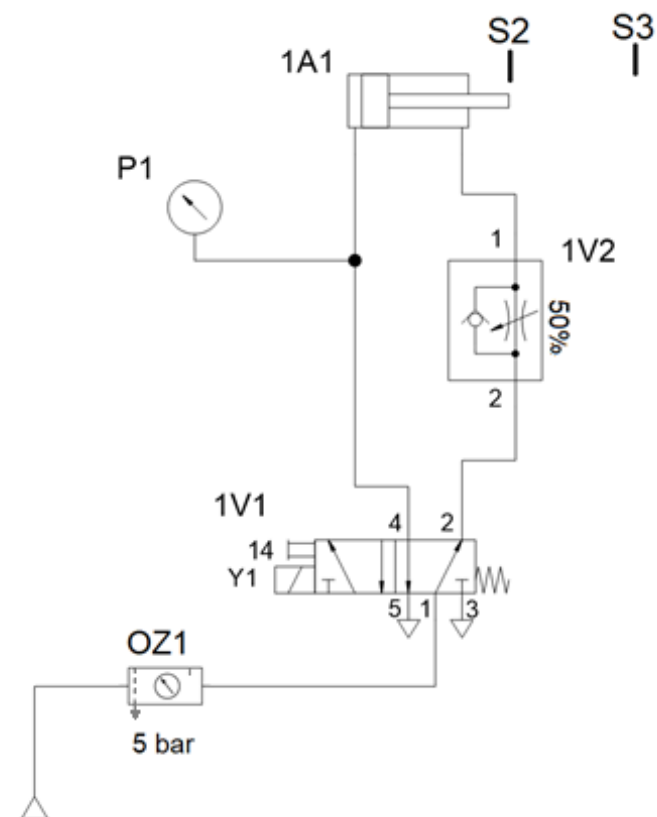
Rysunek 2. Schemat połączeń pneumatycznych
