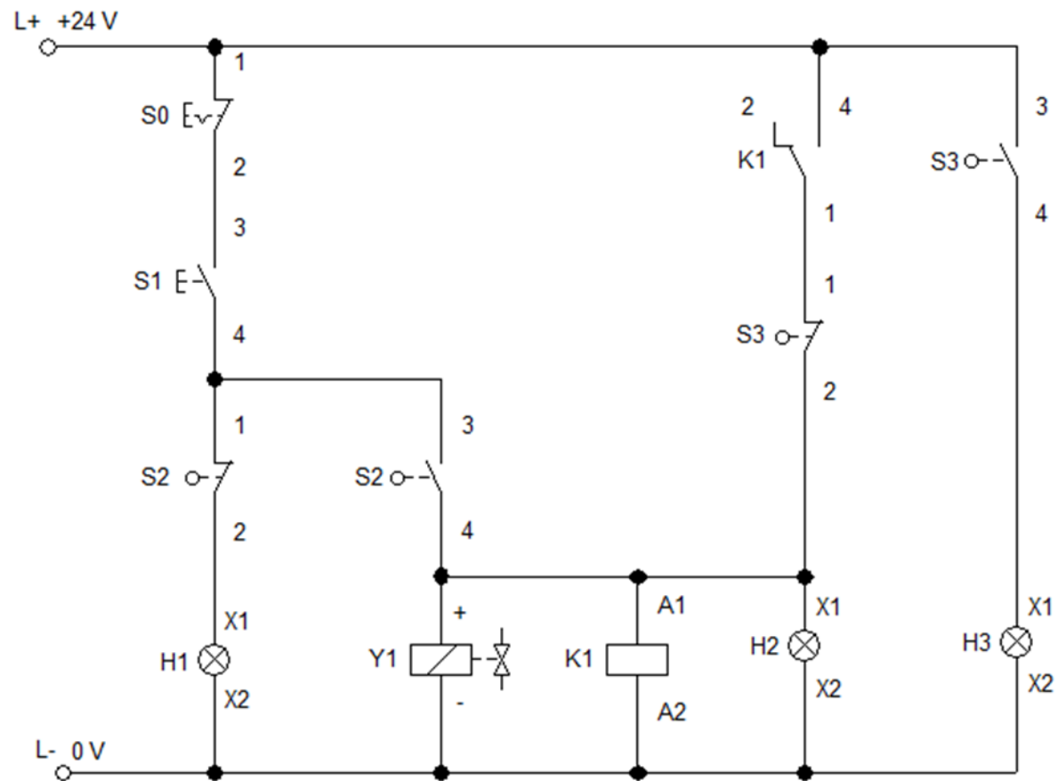
Rysunek 3. Schemat połączeń elektrycznych
