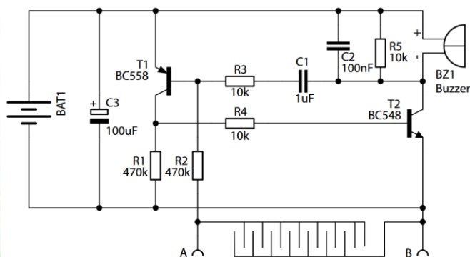
Schemat ideowy
