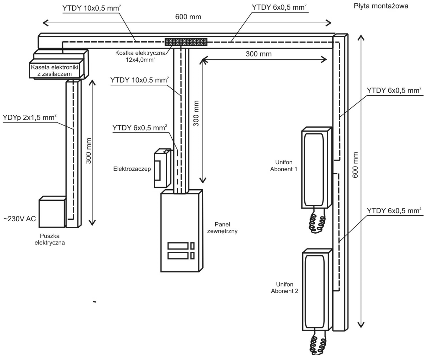
Rysunek 1. Schemat rozmieszczenia elementów instalacji domofonowej.
