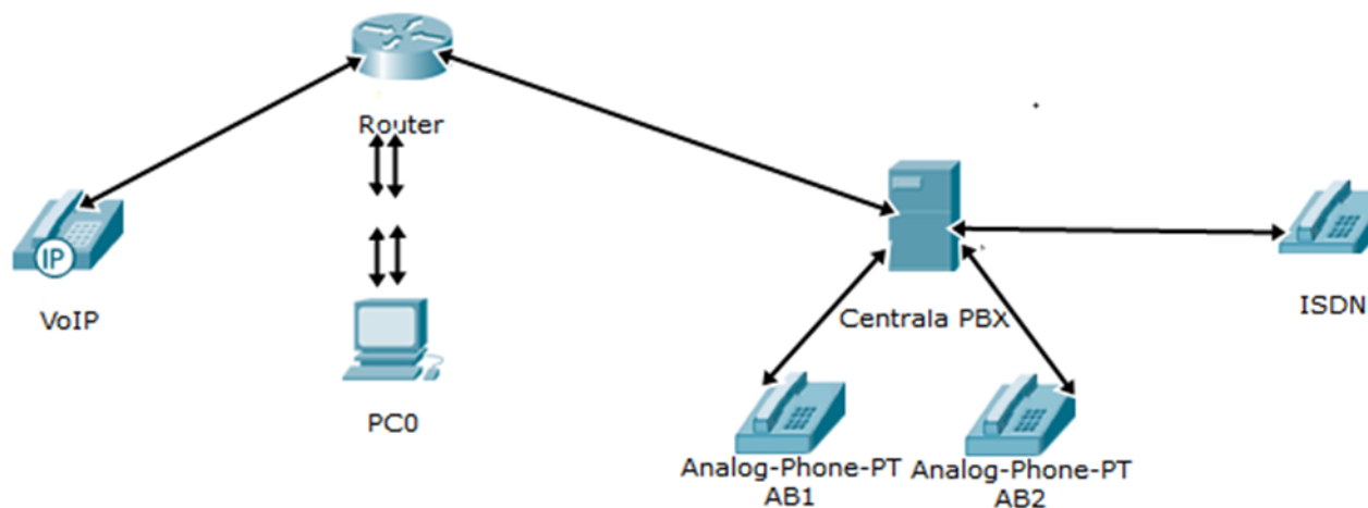
Schemat sieci lokalnej
