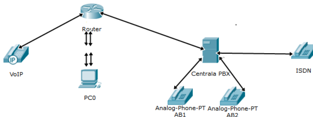
Schemat sieci lokalnej
