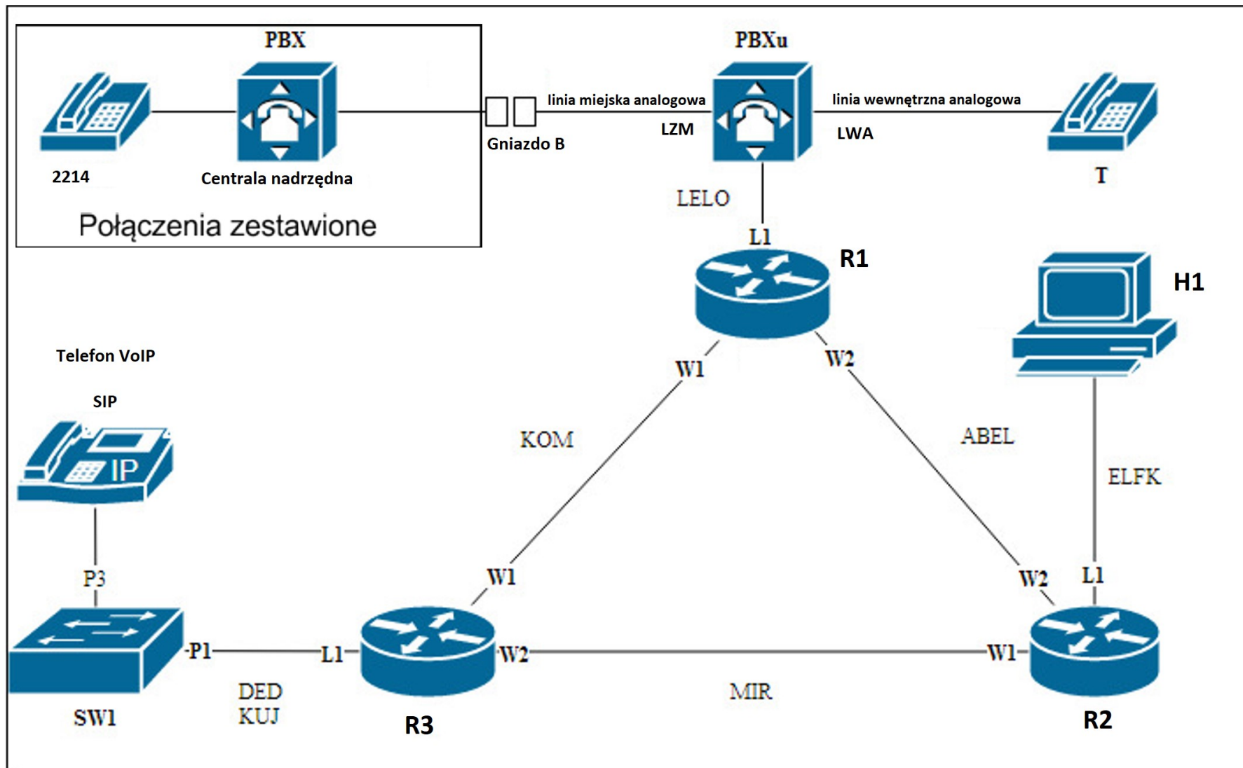
Schemat modernizowanej sieci teleinformatycznej
