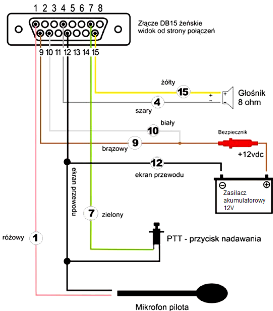
Rysunek 3. Schemat połączeń elementów radiostacji do złącza DB 15 bloku nadawczo-odbiorczego radiostacji XCOM-760 (pominięto listwę zaciskową)
