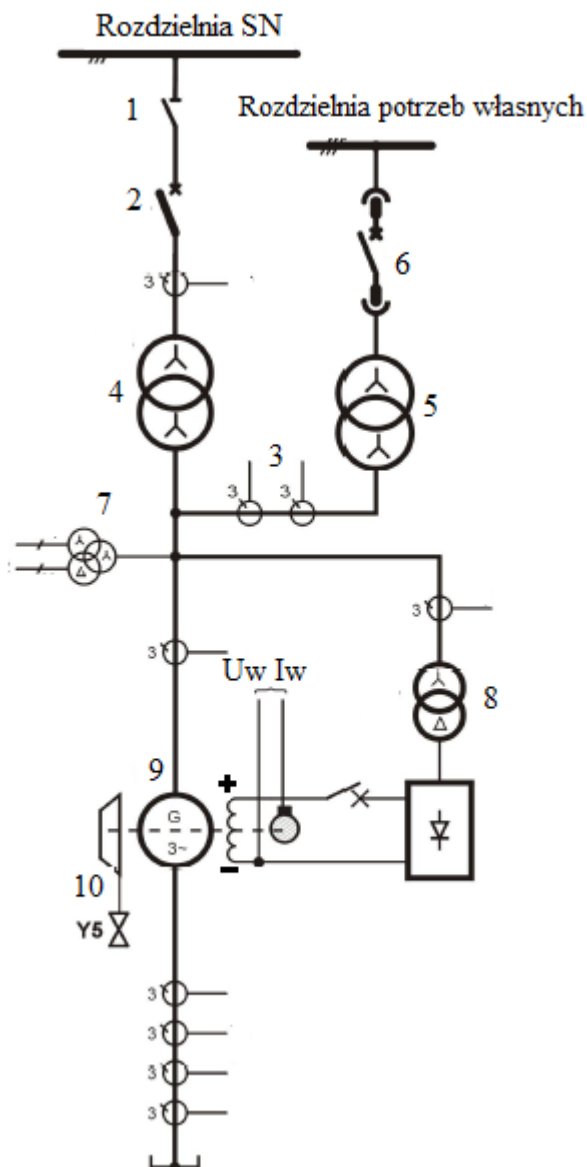
Schemat ideowy połączeń bloku energetycznego
