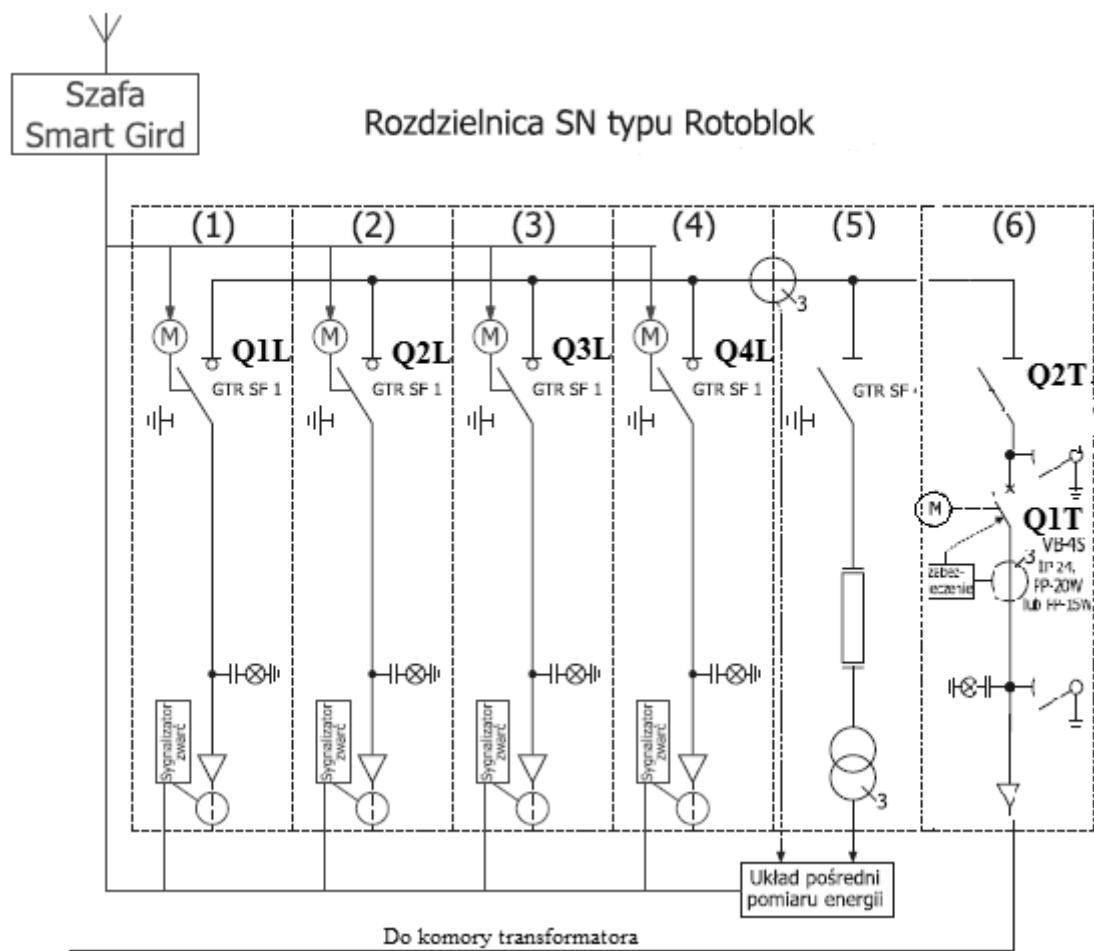
Rys. 3. Schemat rozdzielnicy SN
