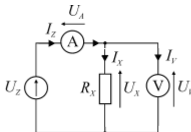
Schemat 4.
