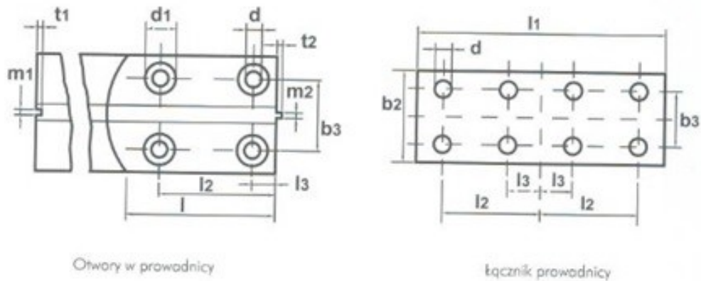
Wymiary przewodnic ciągnionych i łączników w mm
