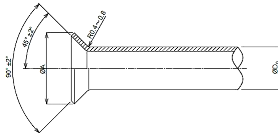
Rysunek 2. Kształt kielichowych zakończeń rurek
