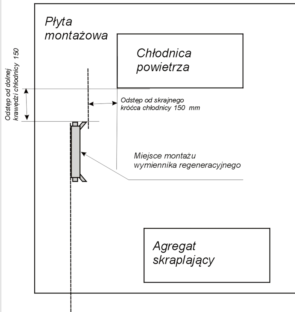
Rysunek 1. Miejsce montażu wymiennika regeneracyjnego
