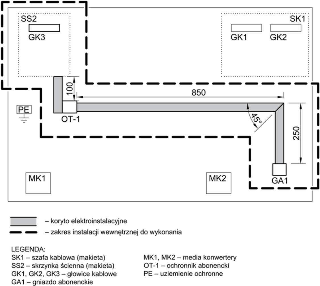
Rysunek 1. Schemat montażowy instalacji abonenckiej
