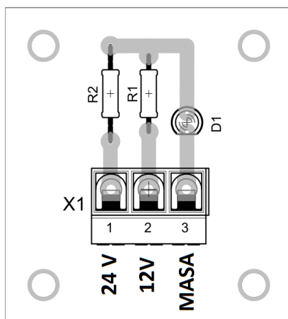
Rys. 4. Schemat montażowy wskaźnika alarmu
