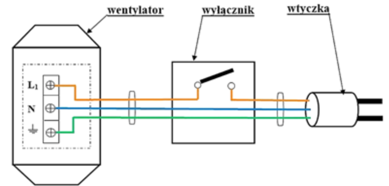
Rysunek 2. Schemat połączeń elektrycznych wentylatora
