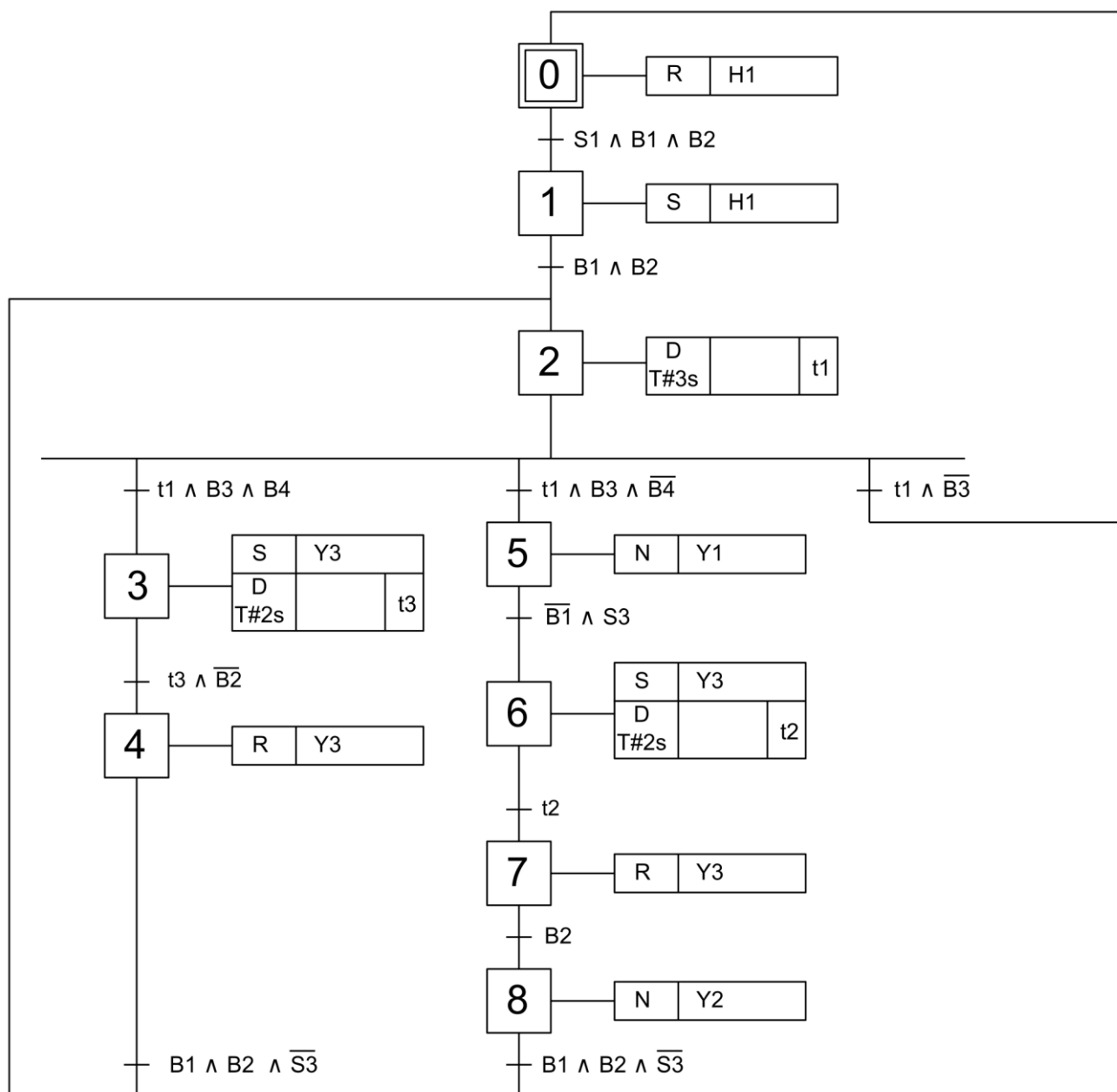
Rysunek 3. Algorytm działania układu rozdzielającego elementy na linii technologicznej*
