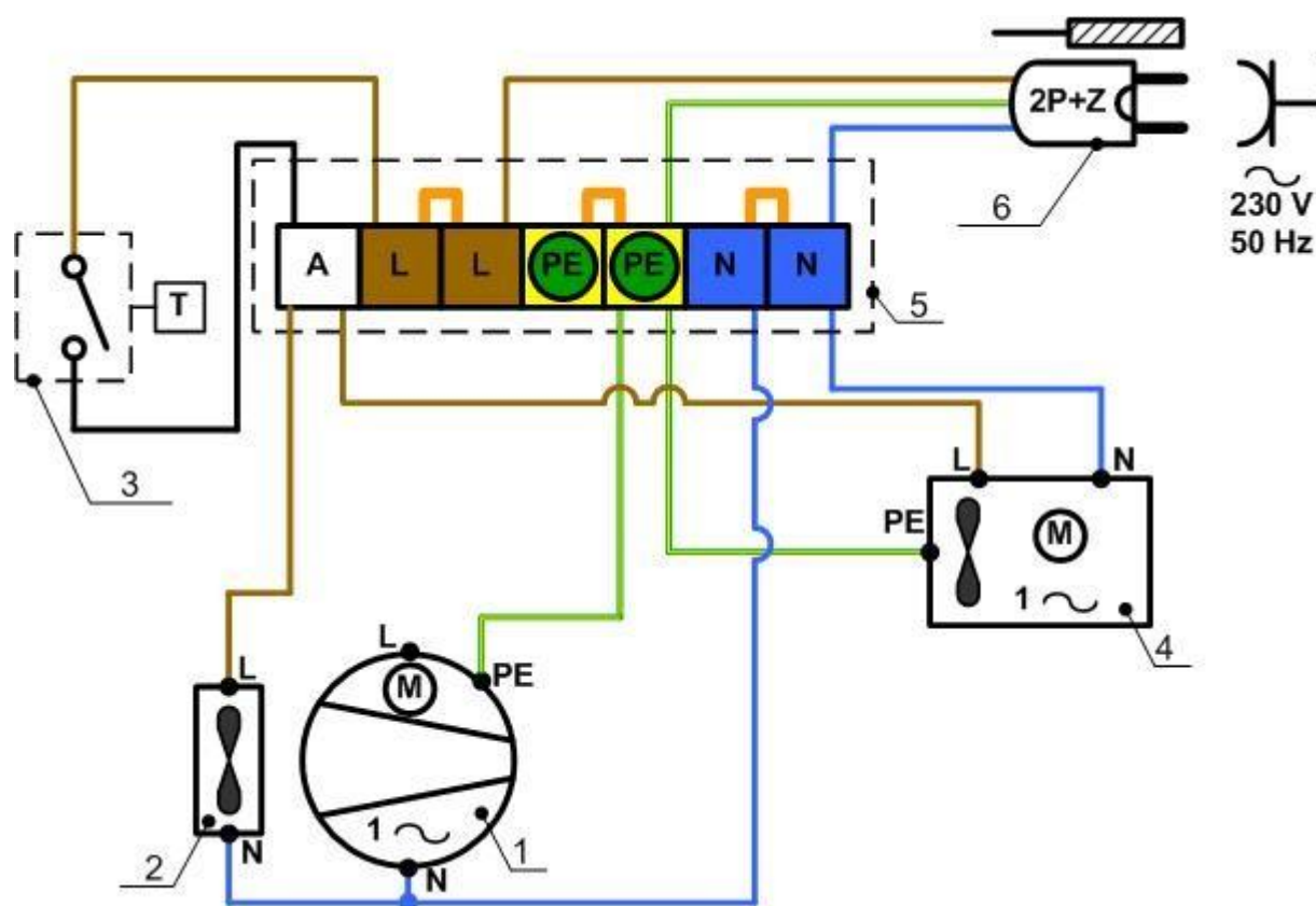
Rysunek 3. Ideowy schemat instalacji elektrycznej przed podłączeniem presostatu
