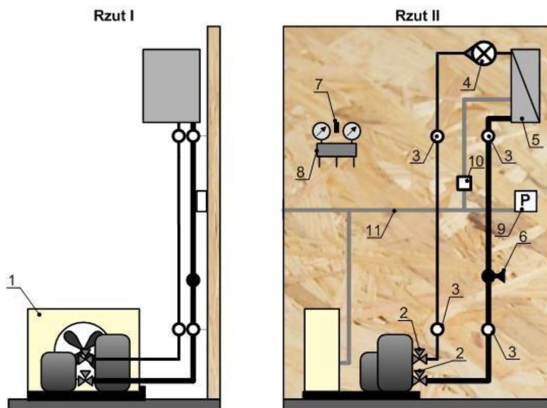
Rysunek 1. Schemat instalacji w układzie chłodniczym przed podłączeniem presostatu
