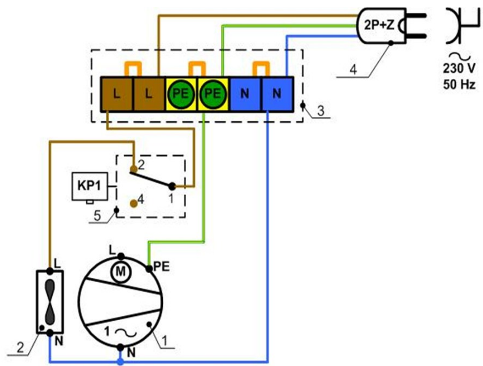
Legenda 1 – Sprężarka; 2 – Wentylator skraplacza; 3 – Puszka podłączeniowa z listwą zaciskową (gwintową); 4 – Wtyczka 2P+Z do gniazda elektrycznego; 5 – Presostat ciśnienia*
