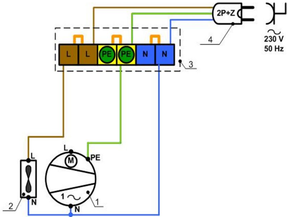
Legenda 1 – Sprężarka; 2 – Wentylator skraplacza; 3 – Puszka podłączeniowa z listwą zaciskową (gwintową); 4 – Wtyczka 2P+Z do gniazda elektrycznego
