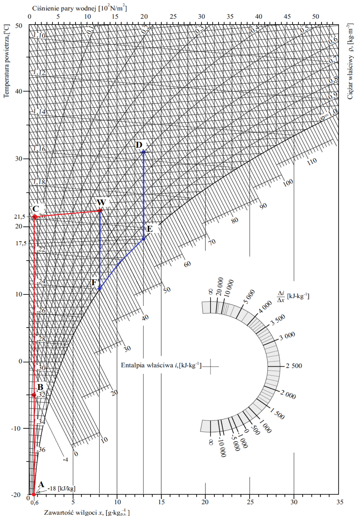
Rysunek 2. Obróbka ciepło-wilgotnościowa powietrza realizowana przez instalację klimatyzacyjną w okresie zimowym i letnim przedstawiona na wykresie Molliera
