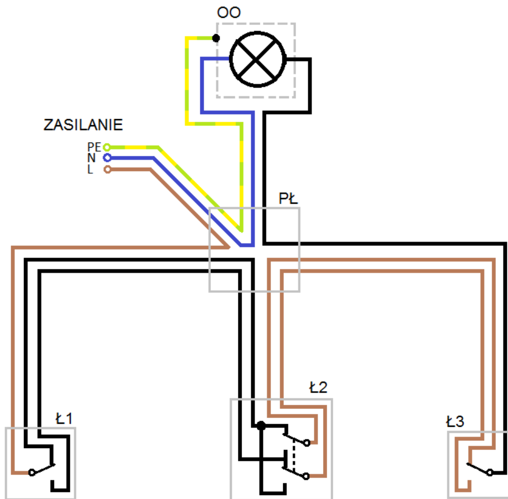
Rysunek 2. Schemat ideowy istniejącej instalacji oświetleniowej korytarza Ł1, Ł2, Ł3 – łączniki instalacyjne, OO – oprawa oświetleniowa, PŁ – puszka łączeniowa
