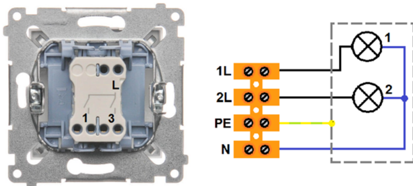
Rysunek 3. Widok łącznika świecznikowego od strony zacisków oraz schemat połączeń żyrandola
