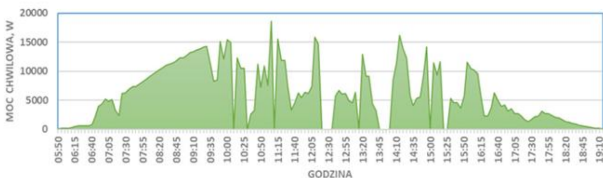
Rysunek 1. Wykresy mocy chwilowej drugiej instalacji fotowoltaicznej w dniach 28 lutego i 11 kwietnia
