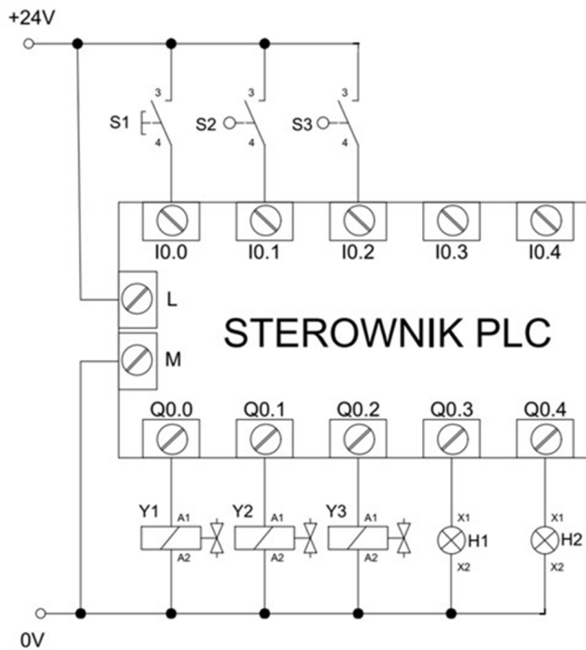
Rysunek 2. Schemat połączeń elektrycznych w układzie elektropneumatycznym
