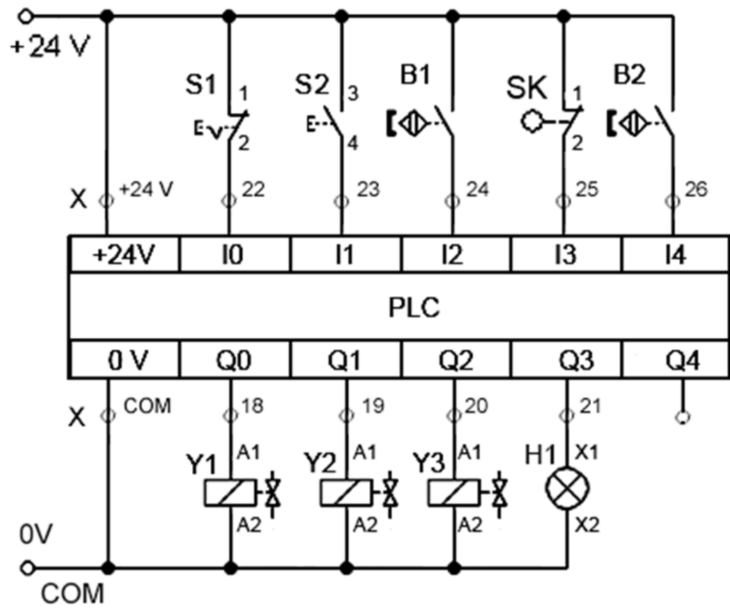
Rysunek 3. Schemat układu elektrycznego
