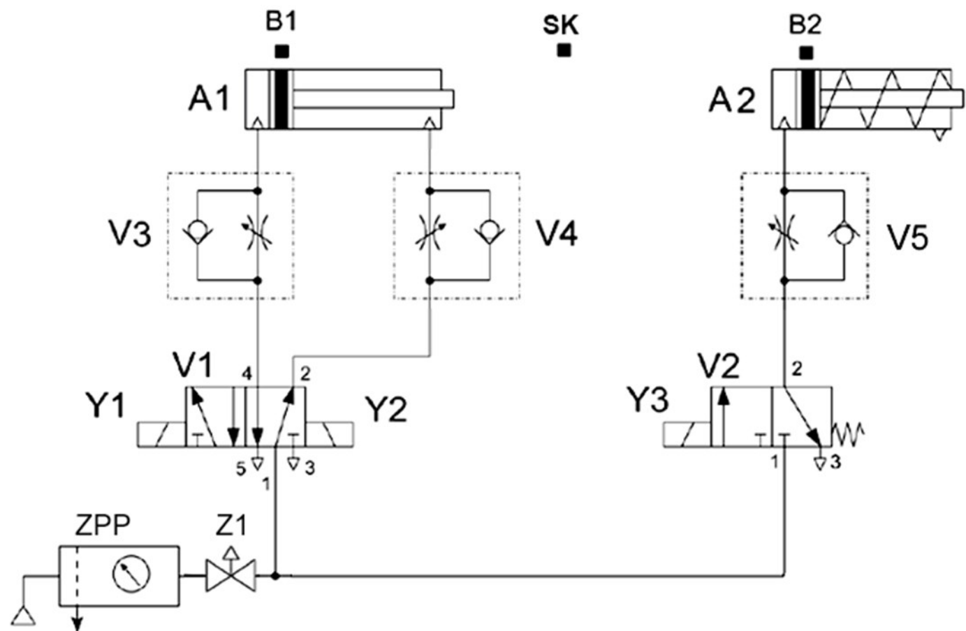
Rysunek 2. Schemat układu pneumatycznego
