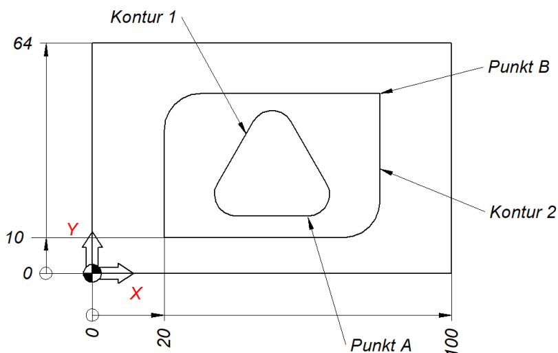
Rysunek 2. Zwymiarowana trajektoria z zaznaczonym układem współrzędnych
