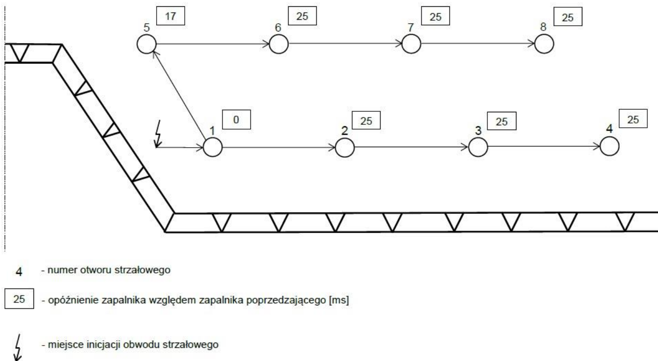
Rysunek 2. Schemat inicjacji sieci strzałowej
