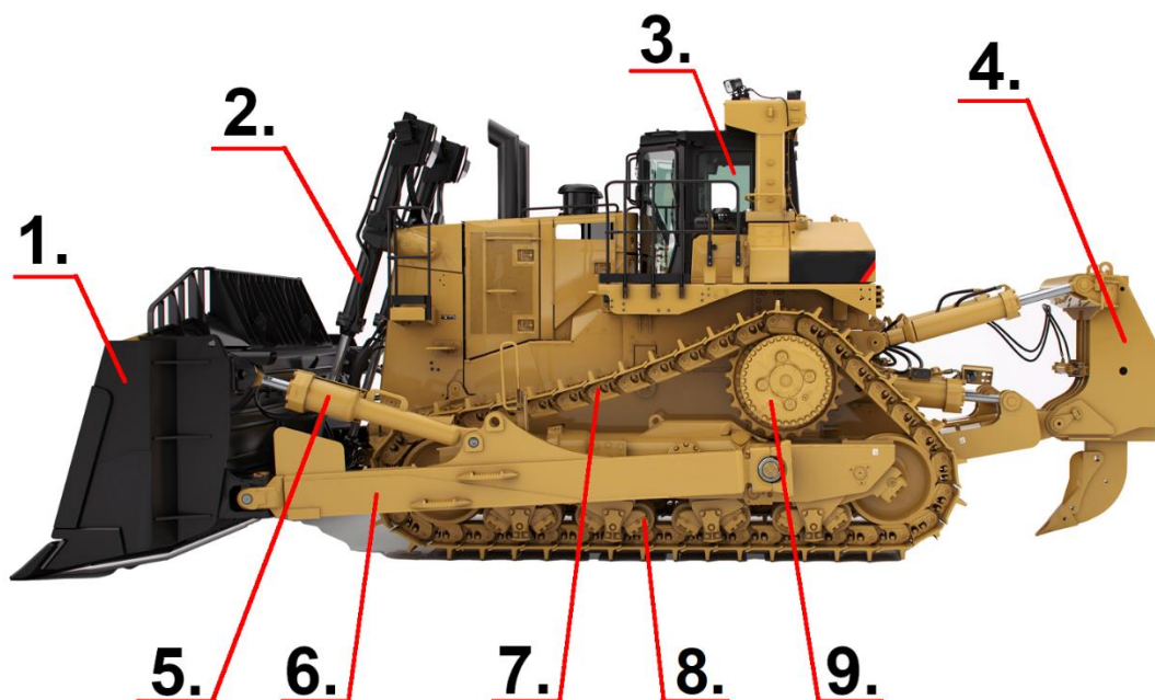
Rysunek 1. Spycharka
