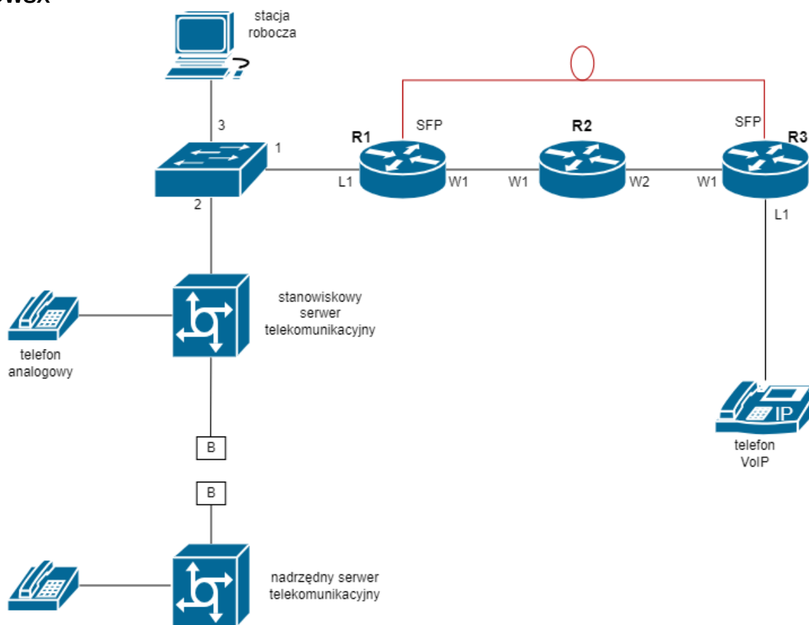
Schemat sieci teleinformatycznej
