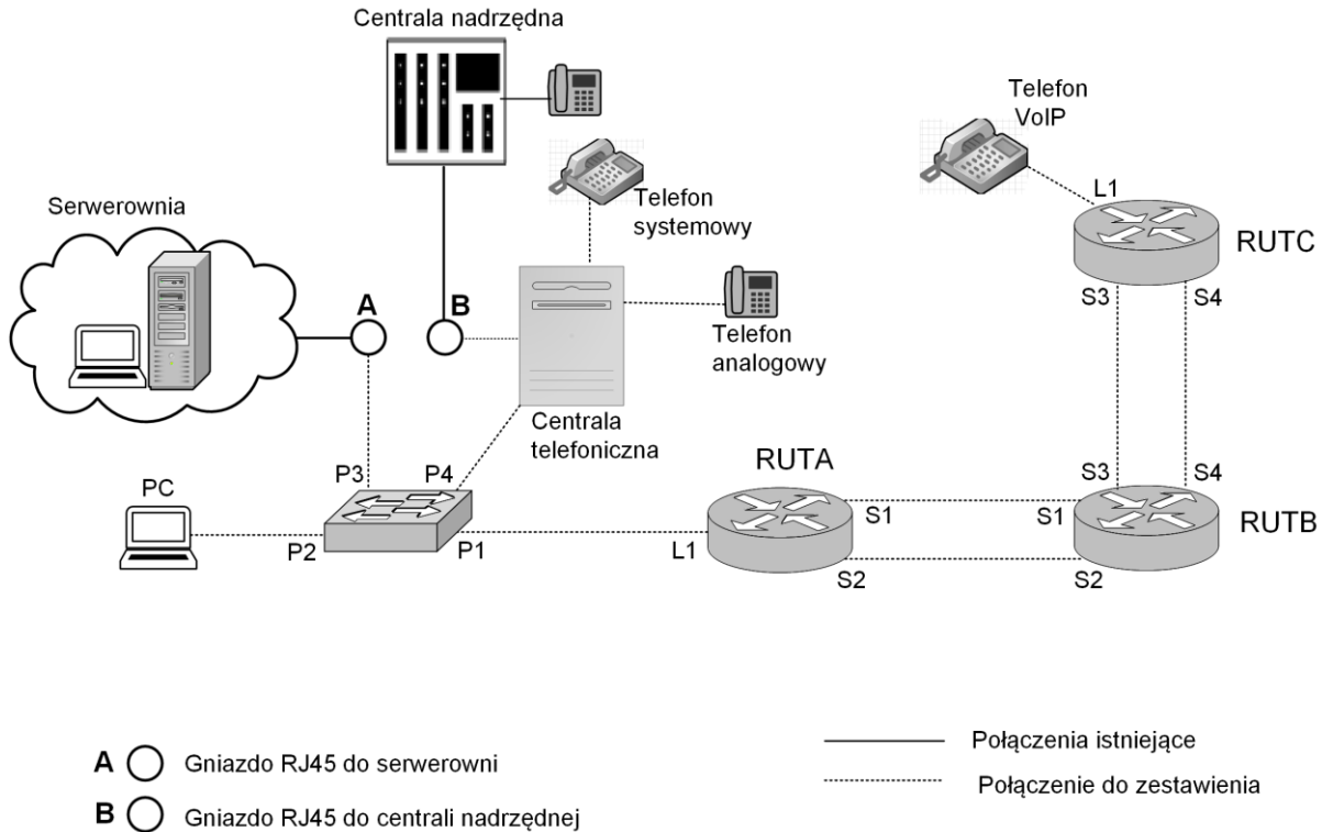
Rys. 1. Schemat usytuowania urządzeń w sieci telekomunikacyjnej
