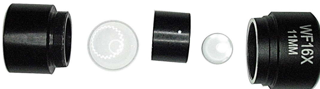
Rys. 2. Okular mikroskopowy o powiększeniu 16 x w rozbiorze na części
