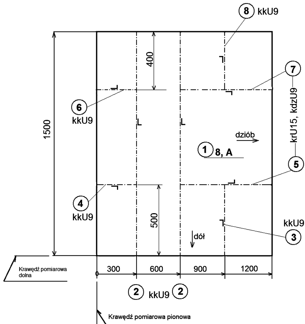
Rysunek 1. Przegroda koferdamu
