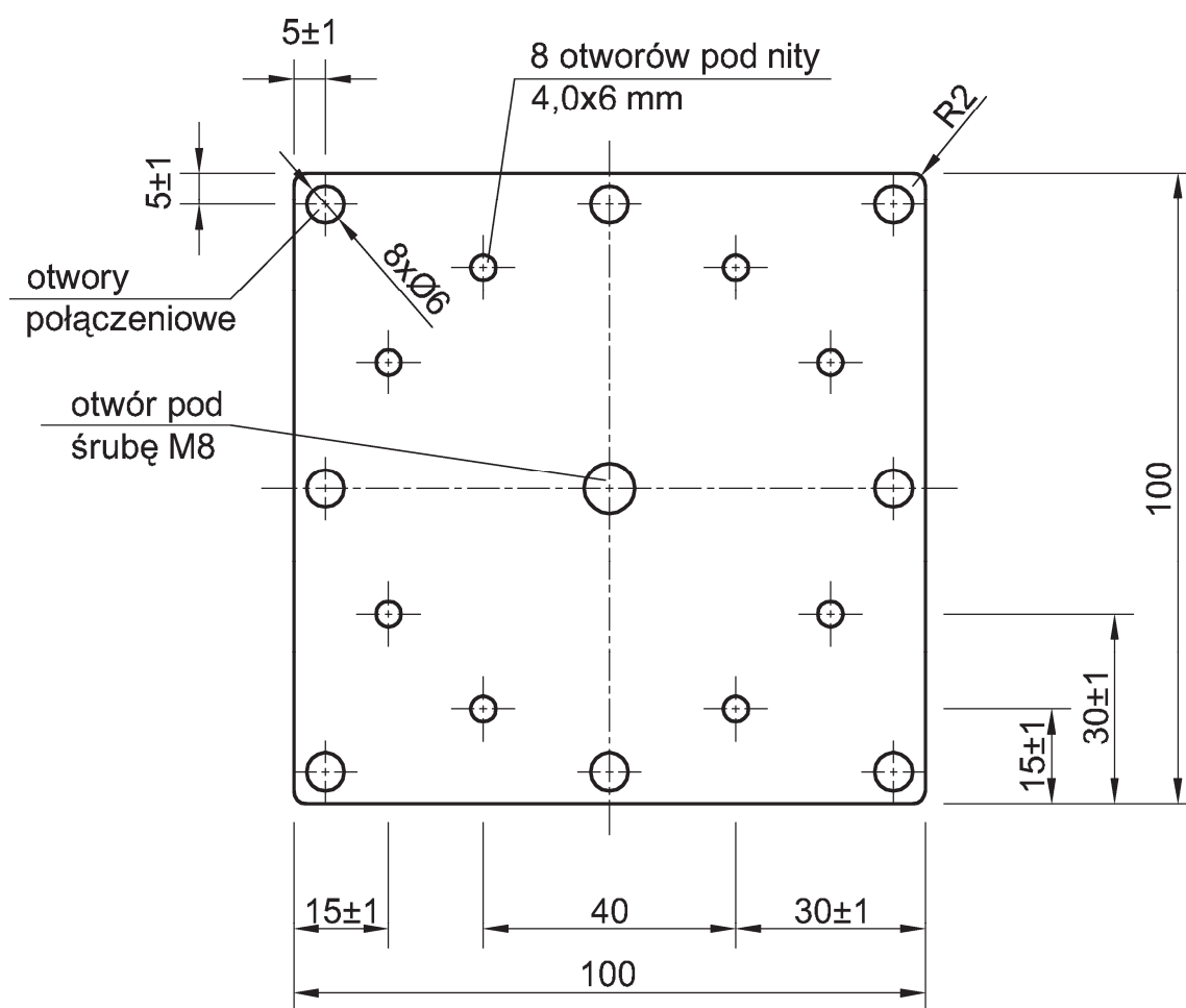
Rysunek 1. Wspornik
